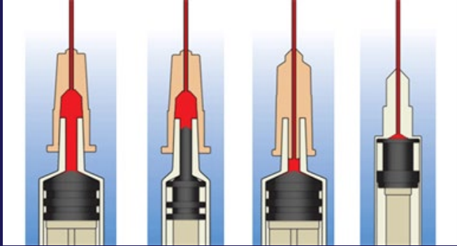
Seringues à corps mort réduit
